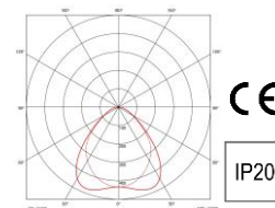
LINEA AL L2 140 MP
