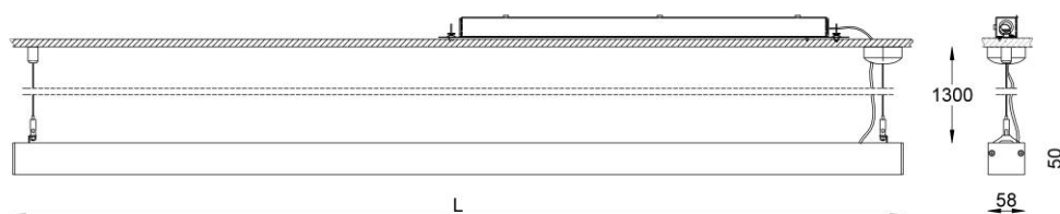
Vaizdas iš šviestuvo šono | Side view
