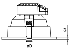
Vaizdas iš šviestuvo šono | Side view
