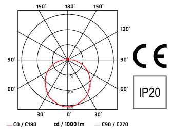
ORBIS S-40 OP 22W 127 lm/W
