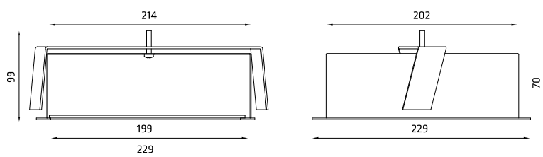
Vaizdas iš šviestuvo šono | Side view
